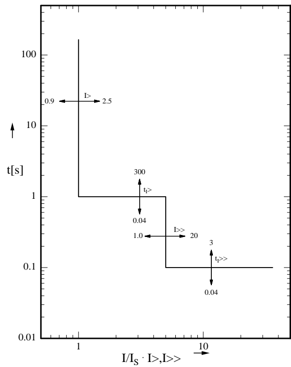
图 4.6: 定时限
