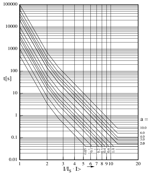
图 4.10: FR-保险丝
