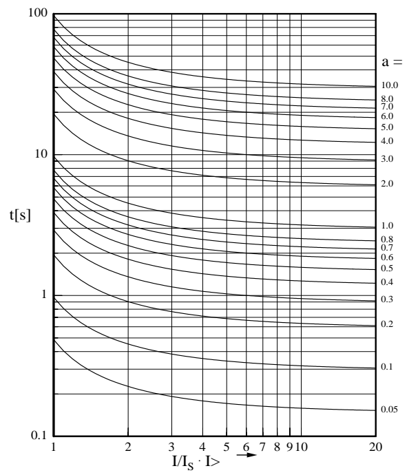
图 4.9: RI-反时限
