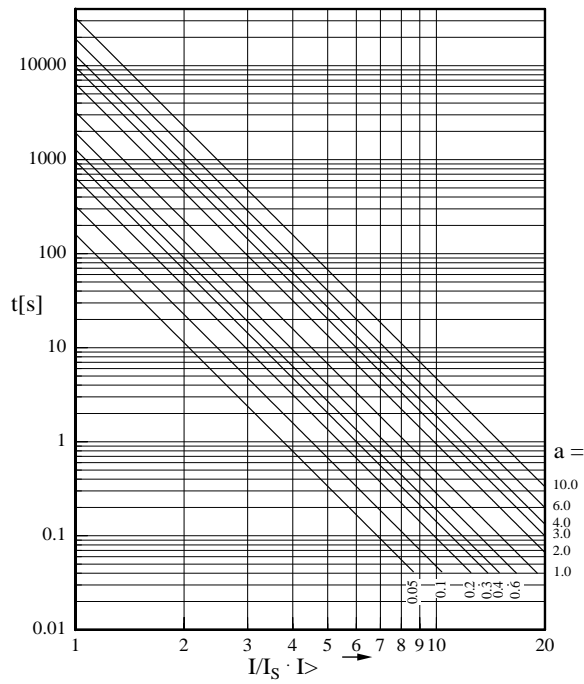
图 4.8: HV 保险丝
