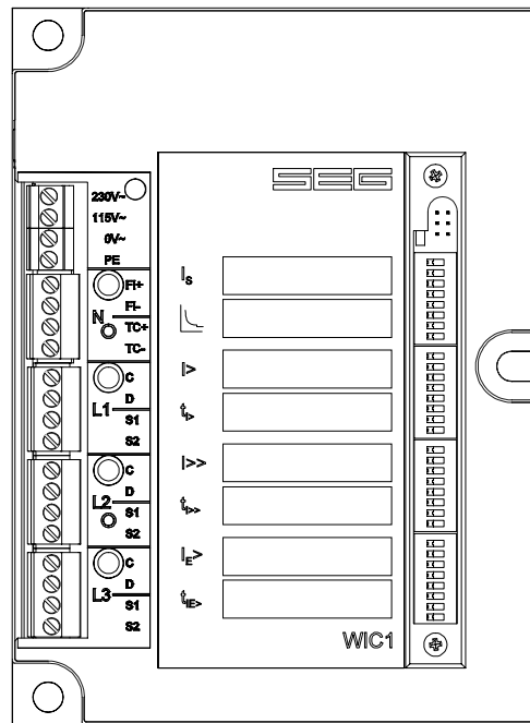
图 3.2: WIC1-2
