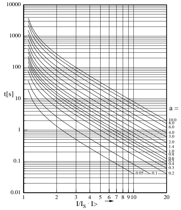
图 4.5: 极端反时限
