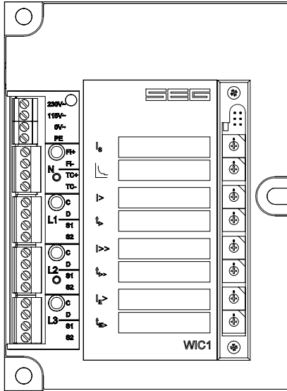
图 3.3: WIC1-3
