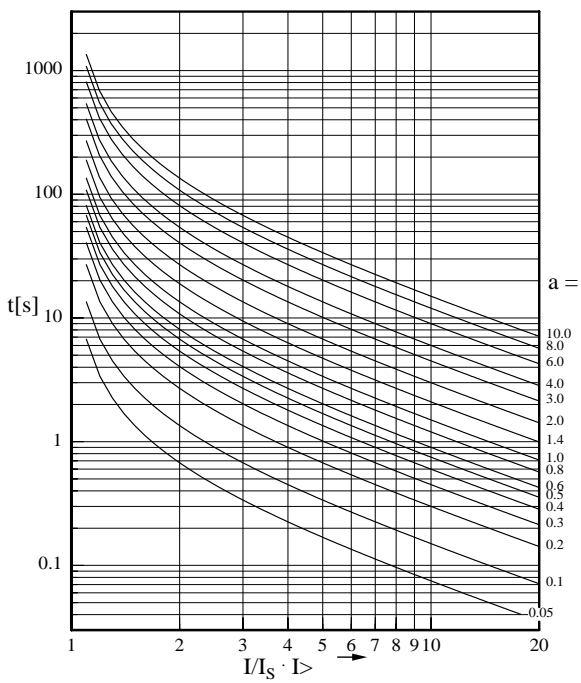
图 4.4: 非常反时限
