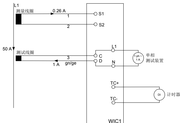
图 6.1: 带 WIC1-W2 型 CT 的单相测试装置(相 L1)的接线
