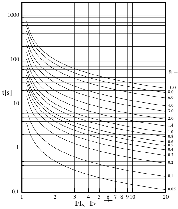
图 4.3: 一般反时限
